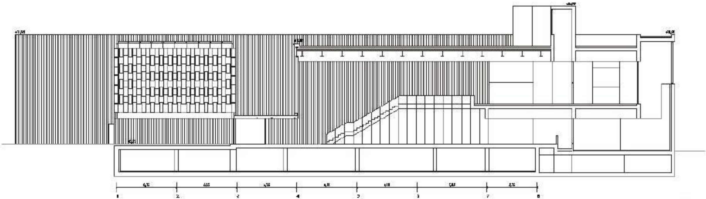
LONGITUDINAL SECTION, LOBBY SECCIÓN LONGITUDINAL POR VESTÍBULO
